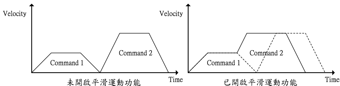
Figure 2.6.4 平滑運動時的速度
