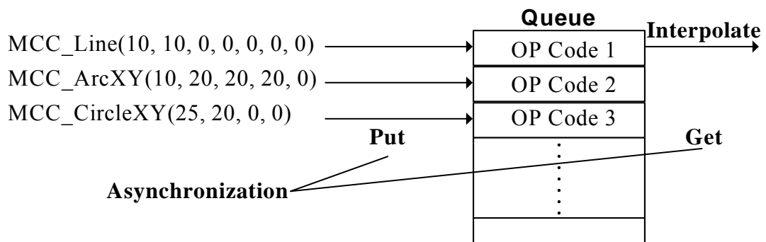
Figure 2.3.2 運動命令緩衝區
