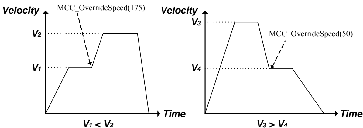
Figure 2.6.6 速度強制
