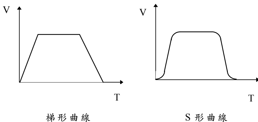
Figure 2.6.3 加減速型式
