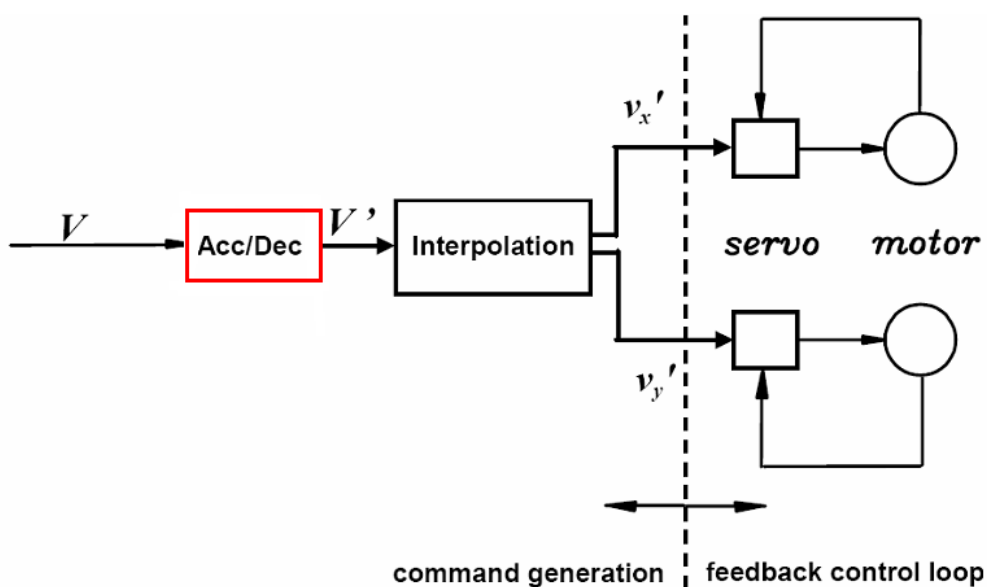
Figure 2.6.9 前加減速模式插值流程
