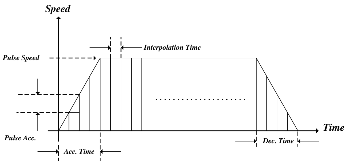
Figure 2.6.7 軌跡規劃設定參數
