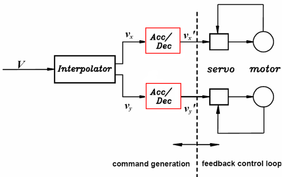
Figure 2.6.8 後加減速模式插值流程
