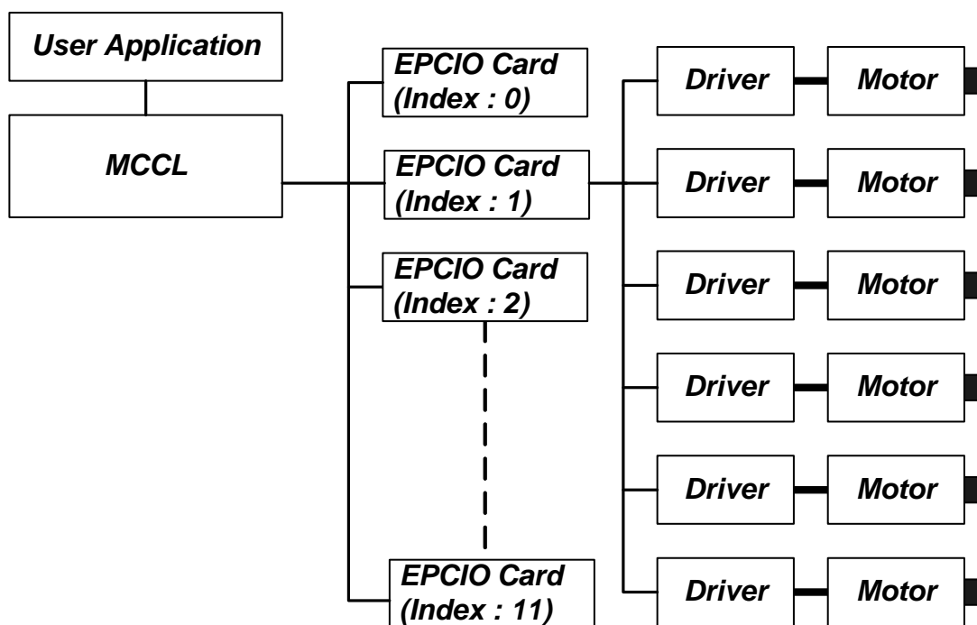
Figure 2.2.2 MCCL 可搭配 12 張 EPCIO 卡
